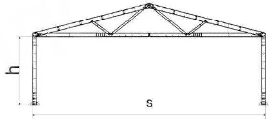
Схема поперечника:
